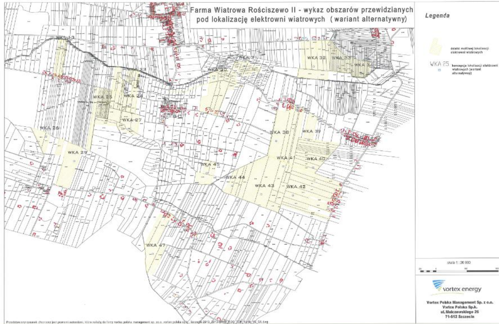
Ryc. 18. Farma Wiatrowa Rościszewo II. Wariant alternatywny.
