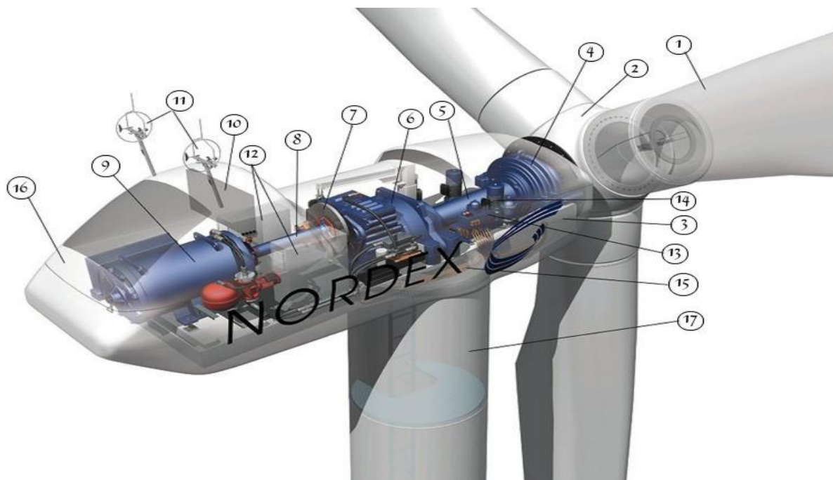
Ryc. 2: Schemat przekroju gondoli siłowni wiatrowej (źródło: www.uwm.edu.pl ).
